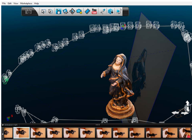
Figura 2. Obtención del modelo 3D por fotogrametría. Disposición de las distintas tomas fotográficas.
