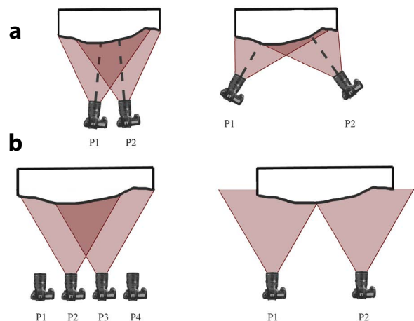
Figura 3. Esquemas correctos (izquierda) e incorrectos (derecha) en las posiciones de las distintas tomas fotográficas.
