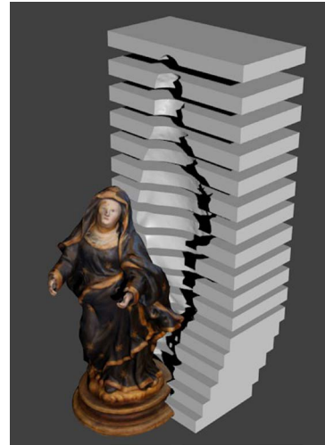
Figura 10. Infografía de embalaje por plantillas rígidas. Desarrollo de la mitad de las distintas partes que comprenderían el embalaje interno.
